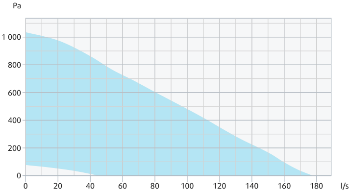
Frånluft - Prestandakurva
