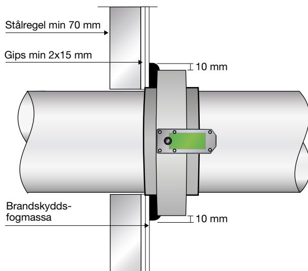
Schaktvägg
